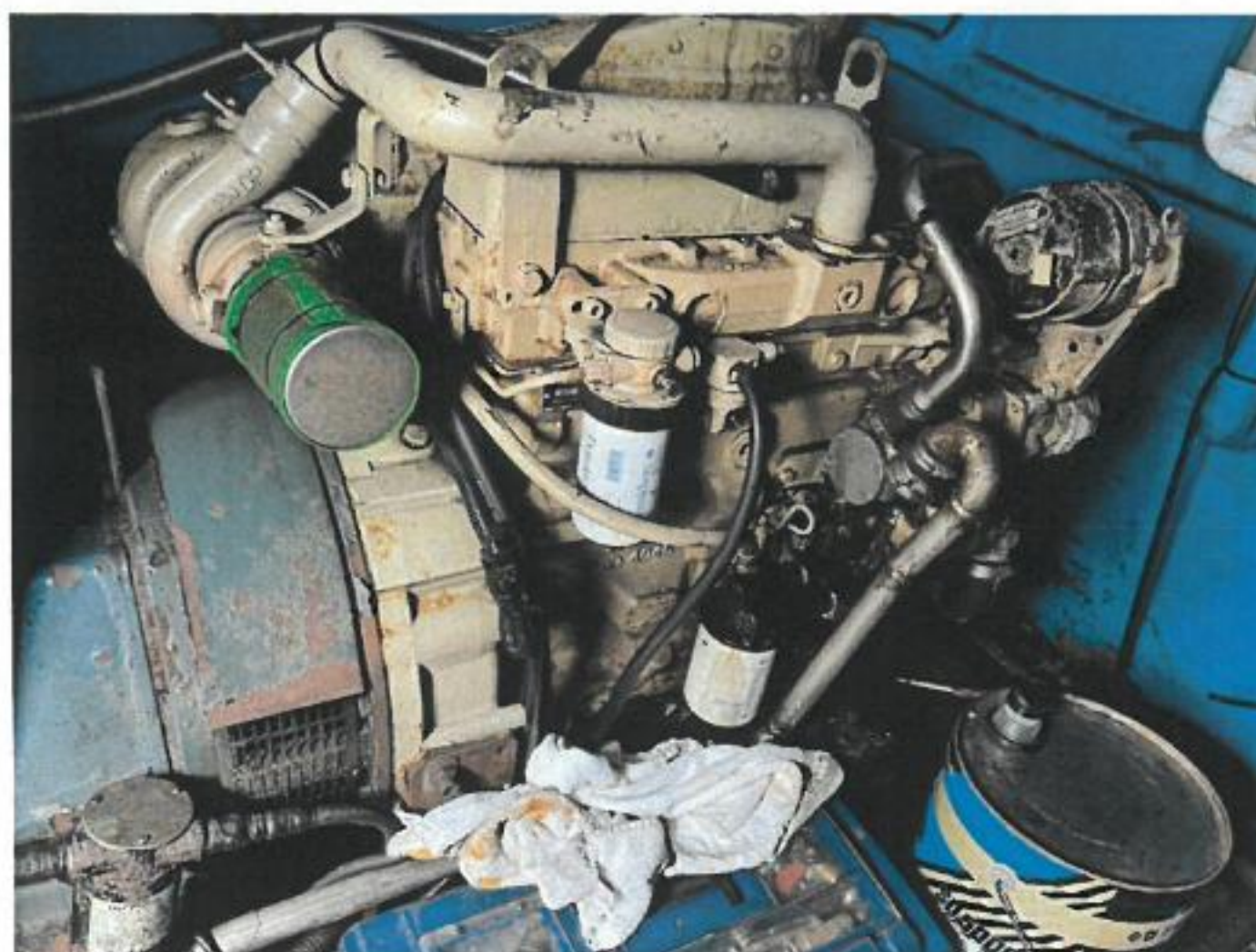
[ 의장품 1)(보조기관) 전경 ]
