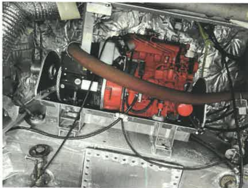
[ 대상물건 의장품 1)(발전기2) 전경 ]
