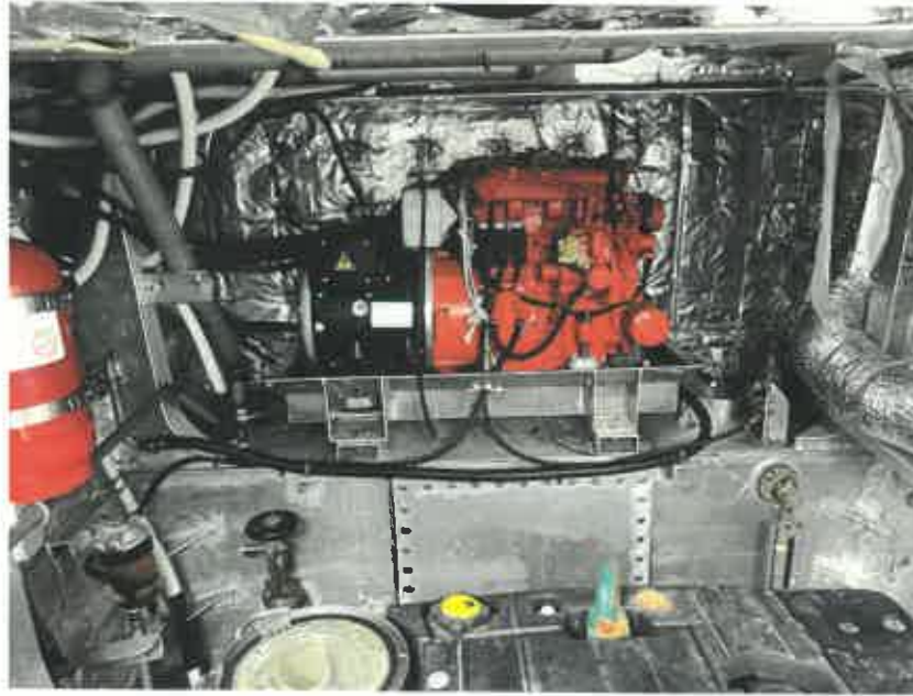
[ 대상물건 의장품 1)(발전기1) 전경 ]
