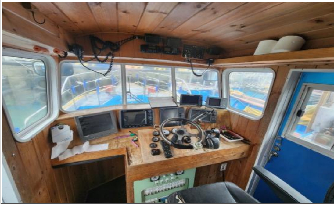
조타실내부
